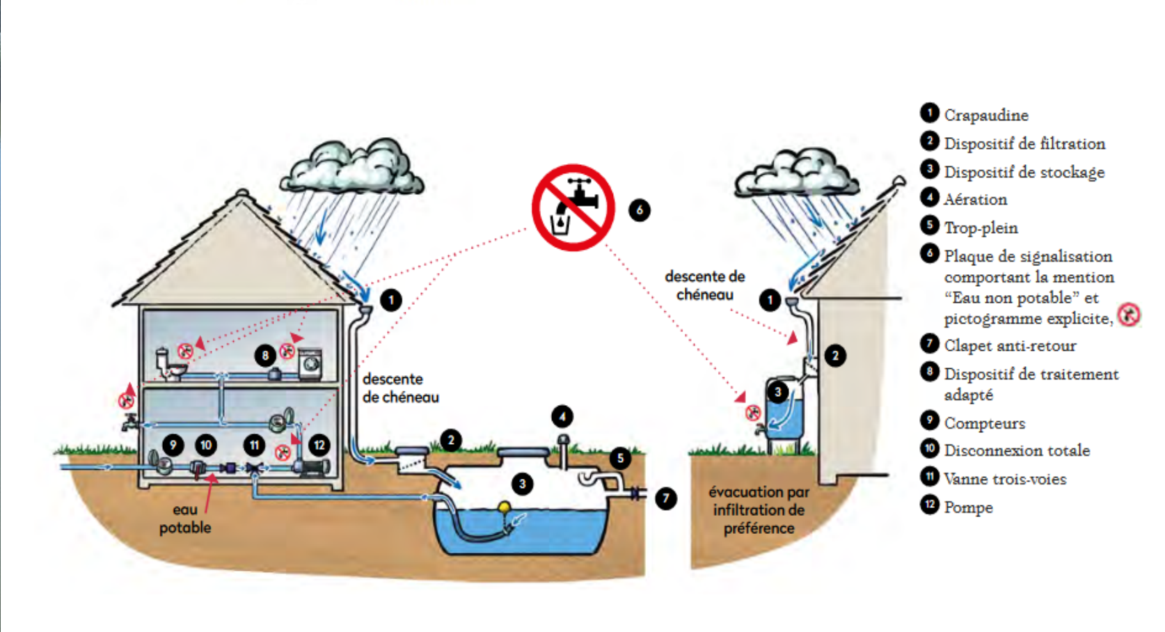
Dispositifs de récupération des eaux pluviales associé à de l'infiltration à la parcelle (logement neuf)
